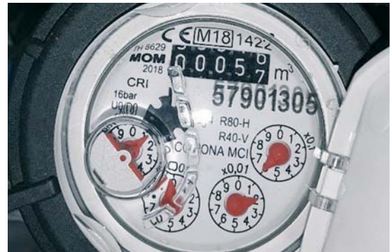
Um den Zählerstand zu erfassen, lesen Sie alle Zahlen, die links von m 3 angezeigt werden, ab. (hier im Beispiel = Zählerstand 57)
