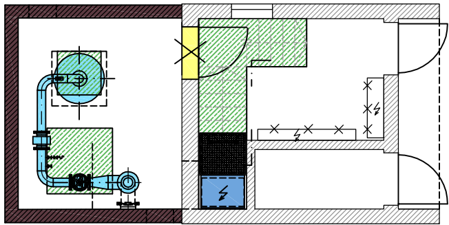
Grundriss Erdgeschoss
